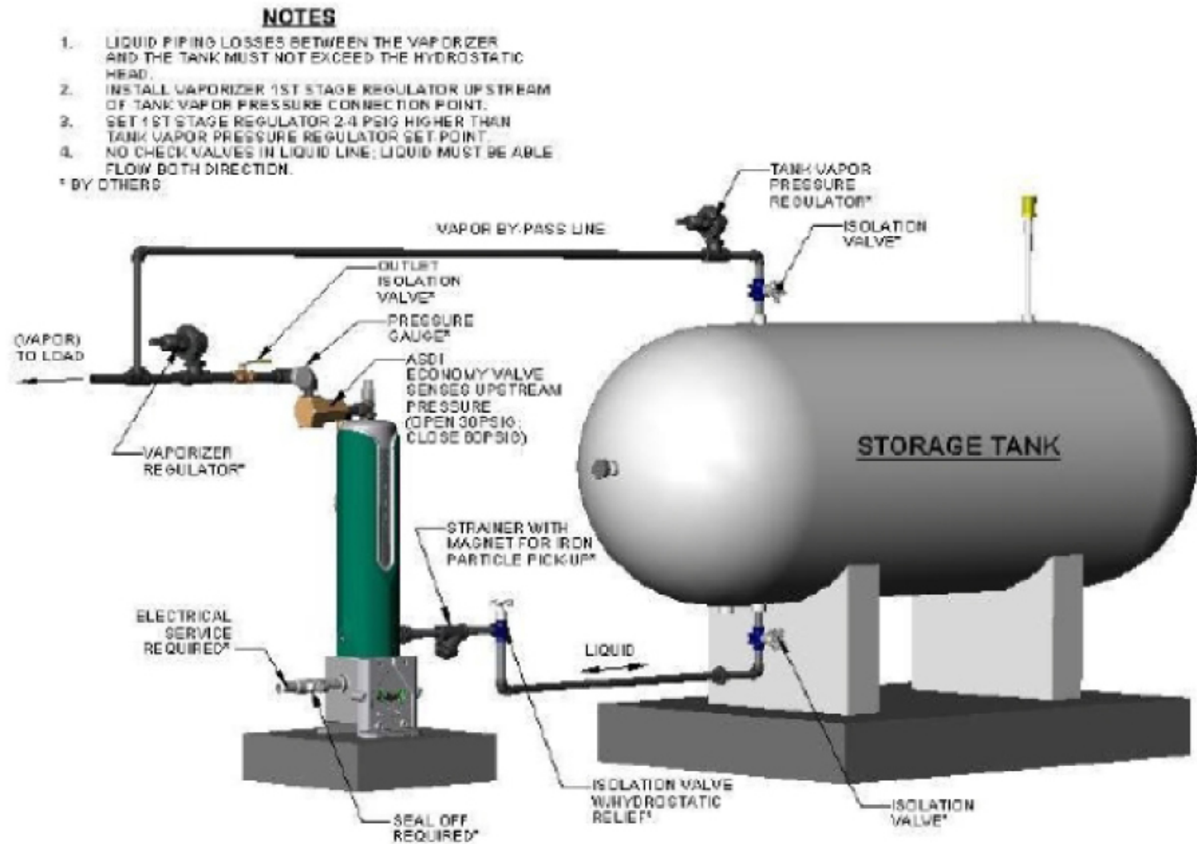
典型安装图/电加热气化器
