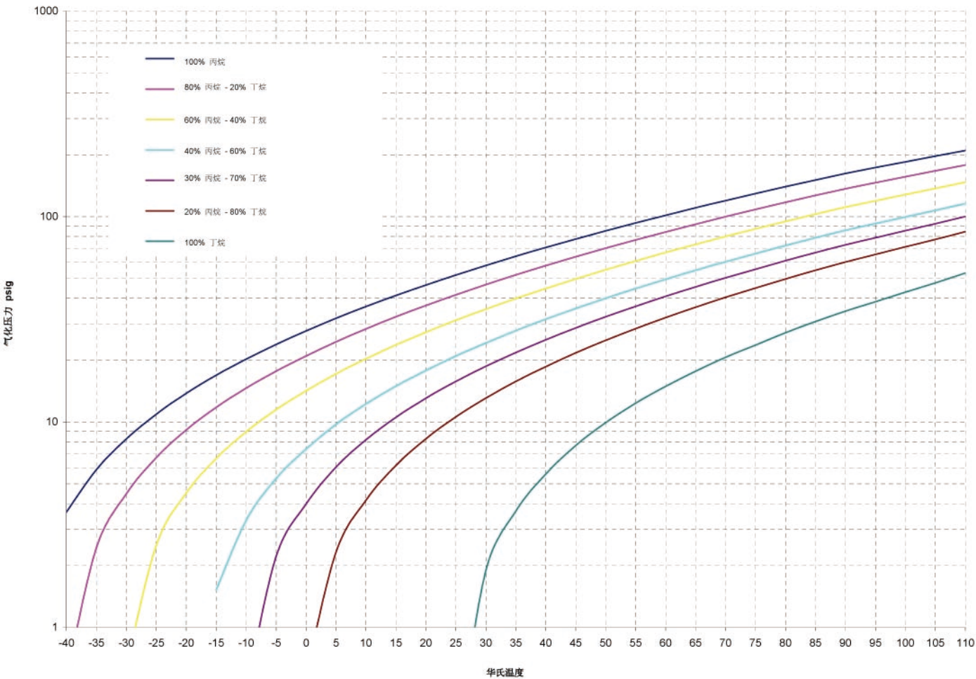
商业丙烷丁烷混合气体 气化压力
